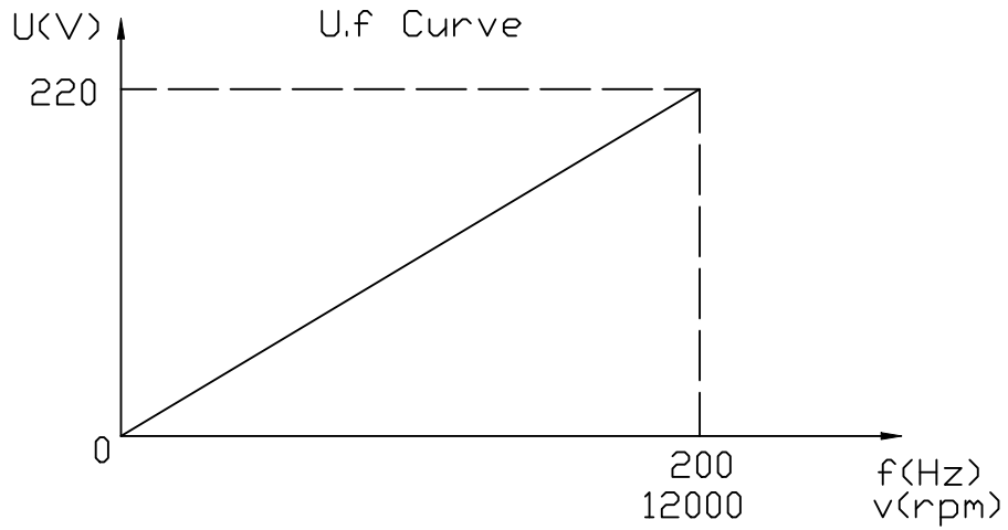
频压曲线
